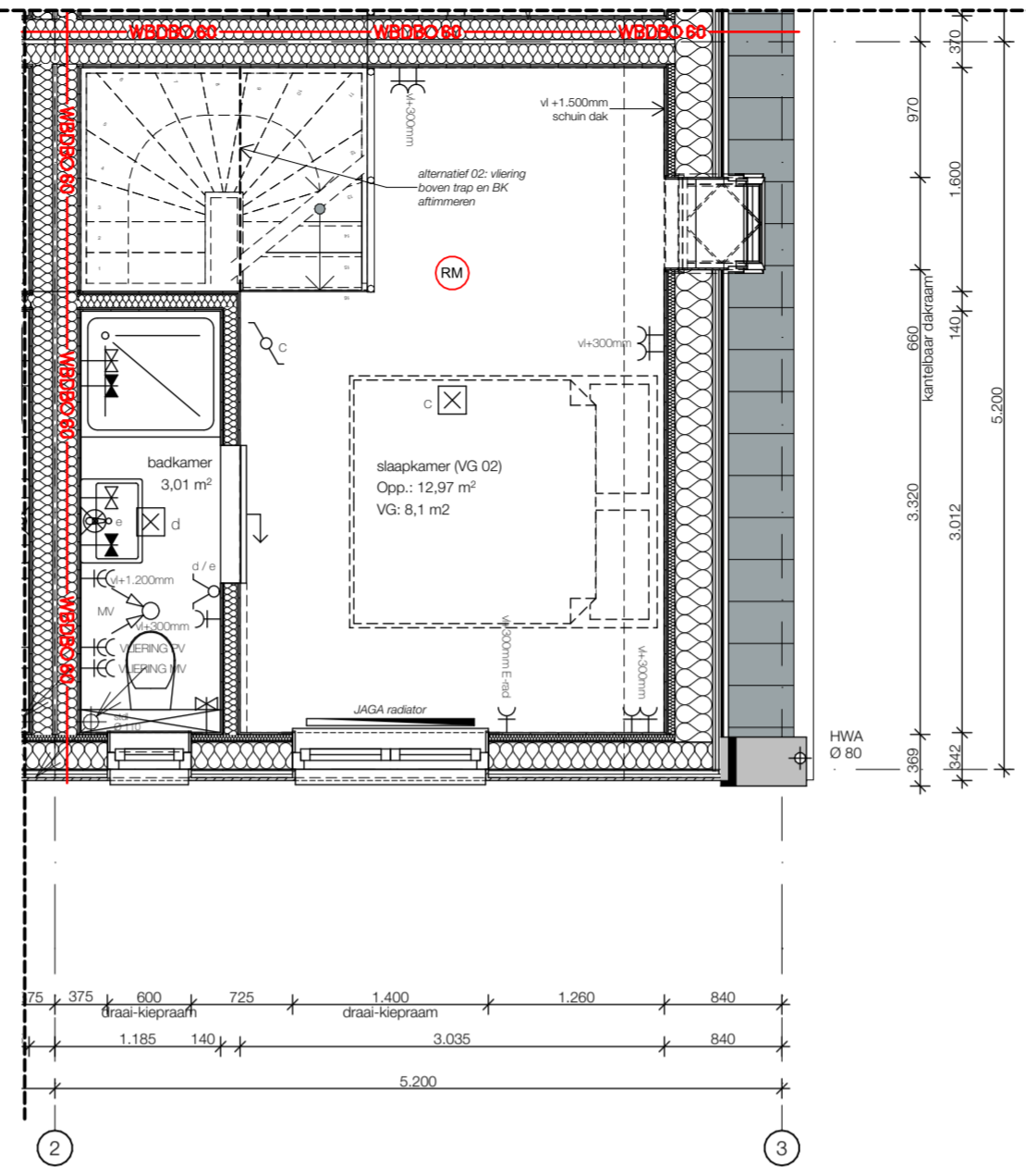
1. 1e verdieping 1:50
