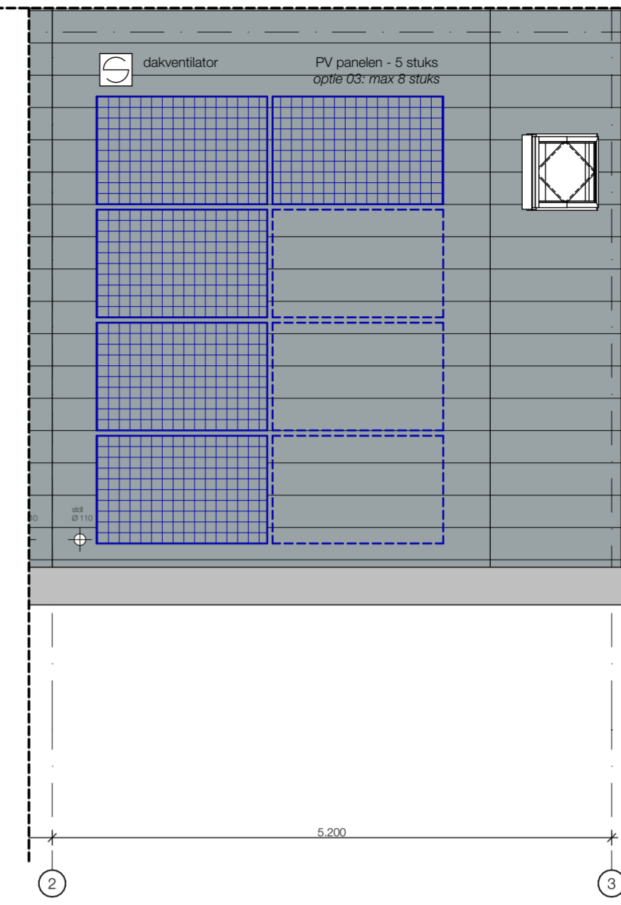
2. Dak overzicht 1:50
