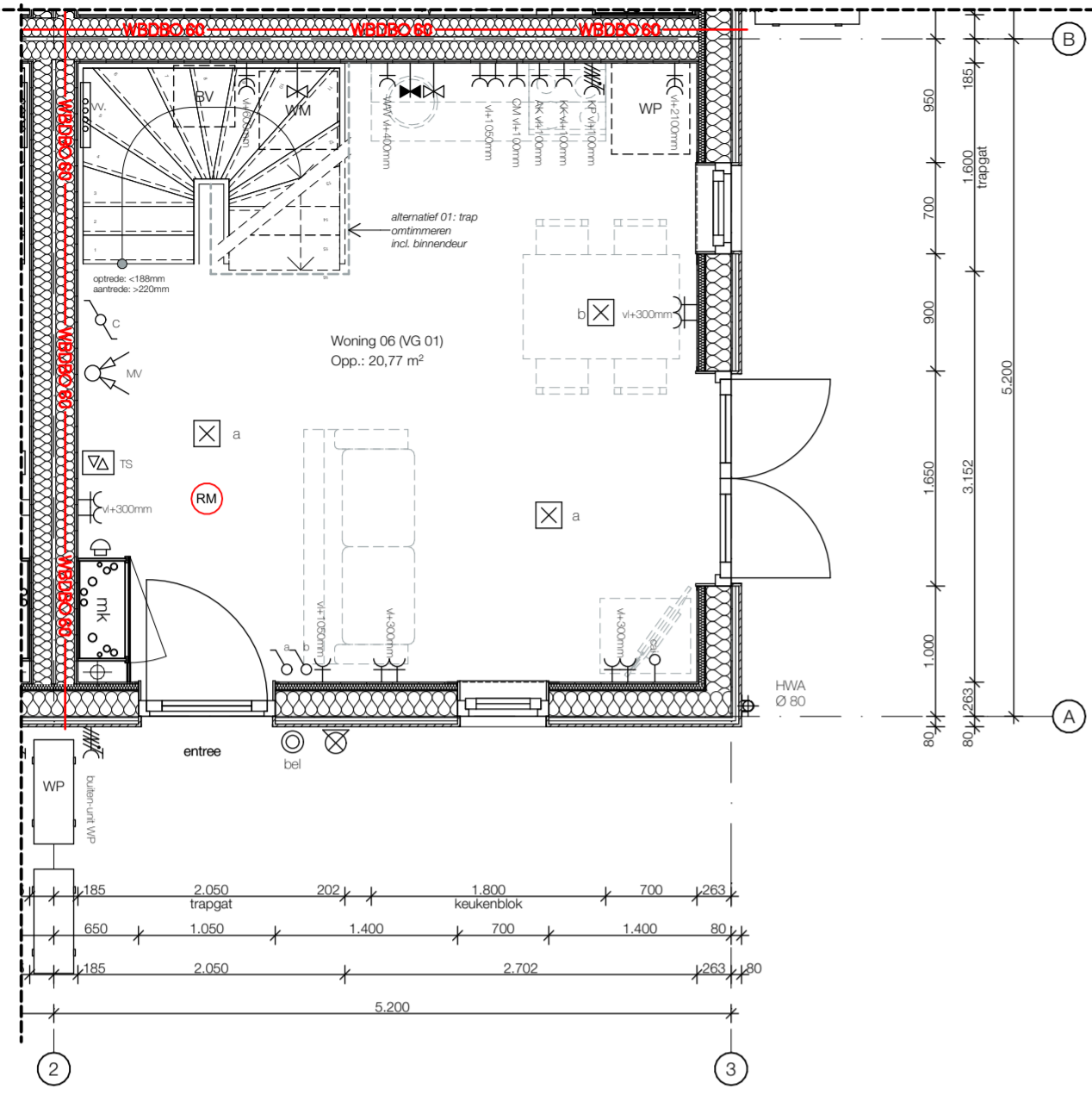
0. Begane grond 1:50
