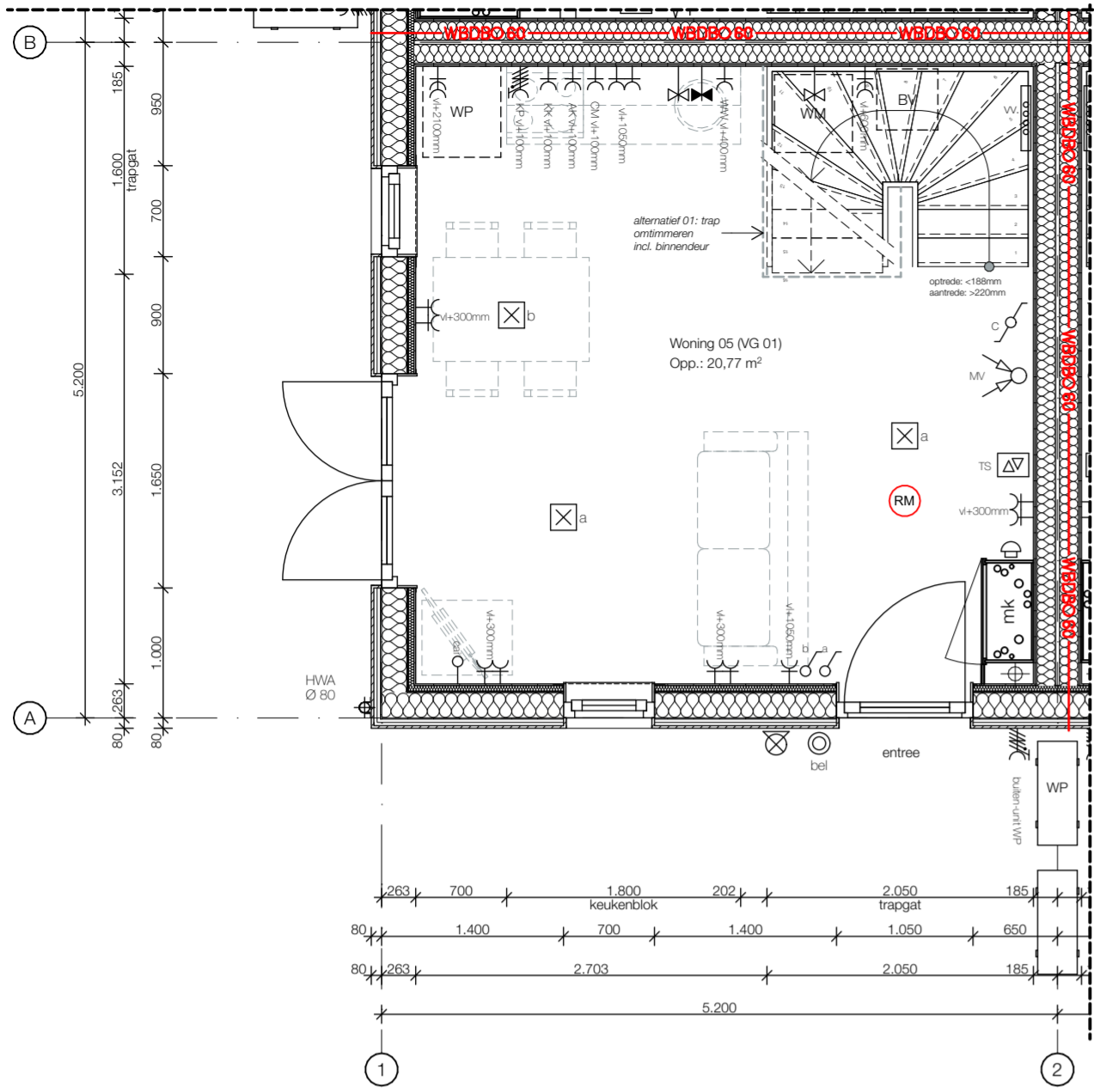
0. Begane grond 1:50
