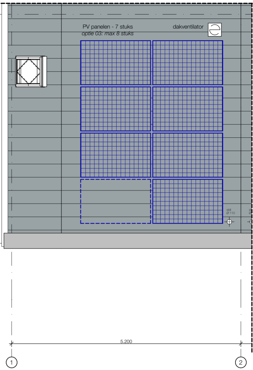
2. Dak overzicht 1:50
