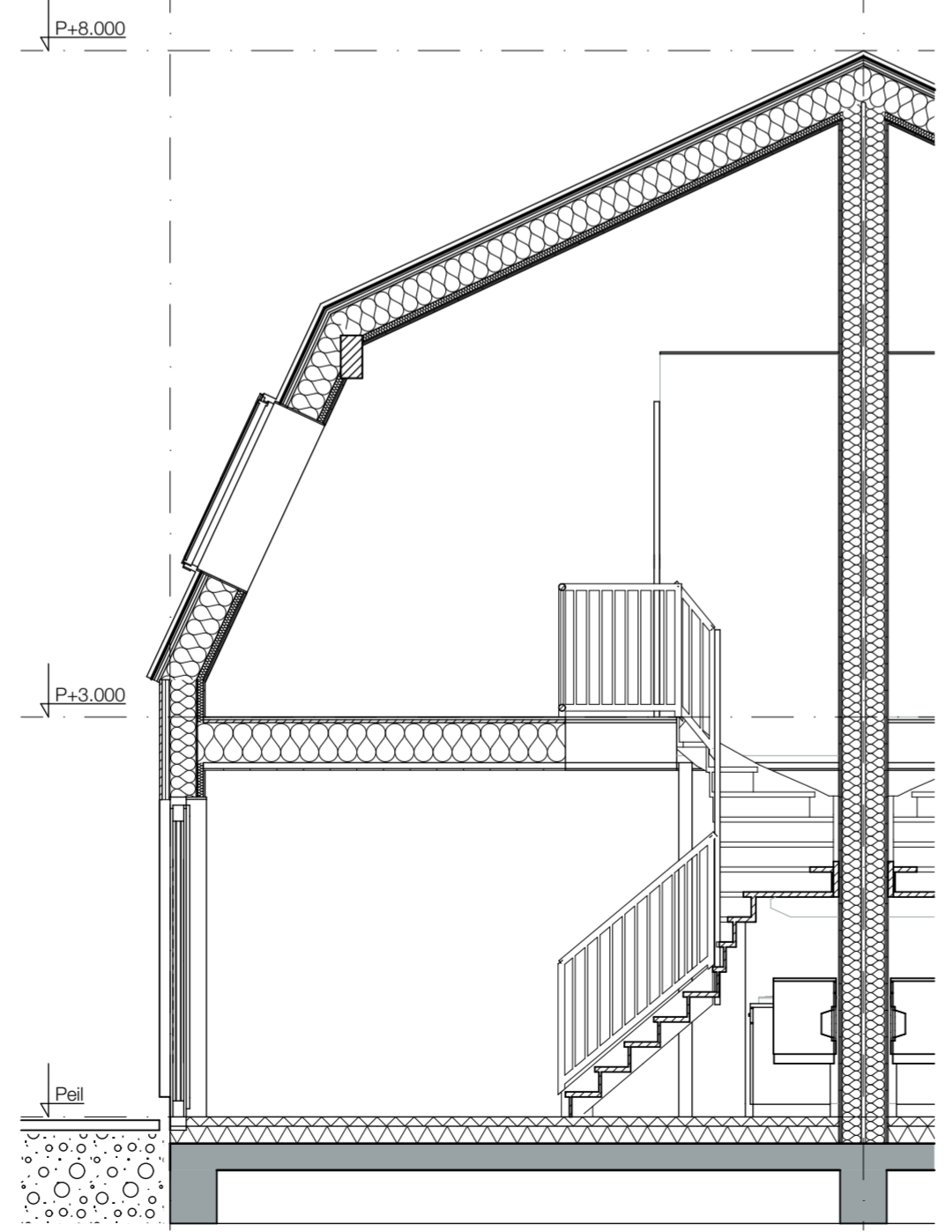
A Doorsnede A-A 1:50
